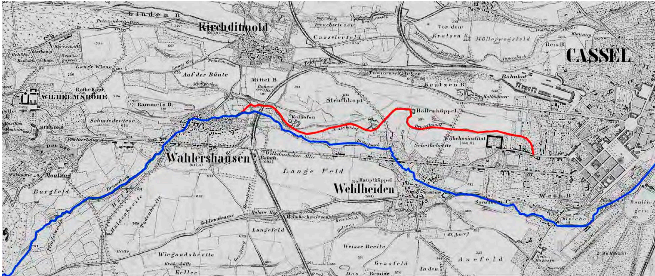
Ausschnitt aus: Kurfürstenthum Hessen. Niveau Karte auf 112 Blättern nach 25000 d. w. G. • Blatt Nr.15: WILHELMSHÖHE • 1859 • nicht maßstabgerecht rot markiert: Druselgraben • blau markiert: Druselbach
